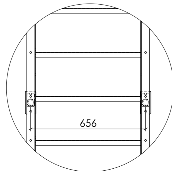
DETAIL AZ SCALE 2 : 25
