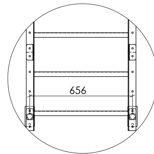
DETAIL BI SCALE 1 : 14
